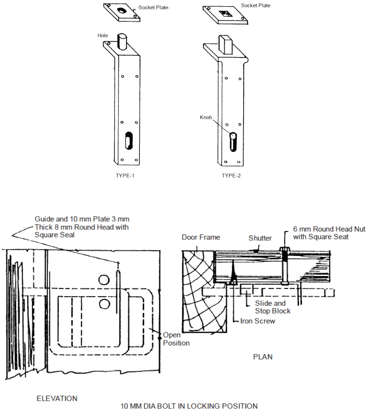
Fig. 14.3 : Flush Bolts
