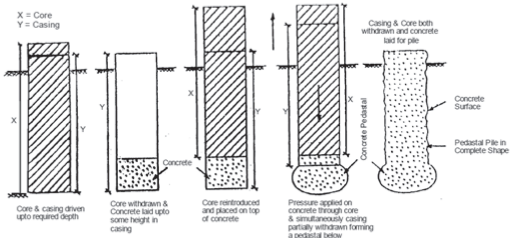
Fig. 20.2 : Pedestal Piles
