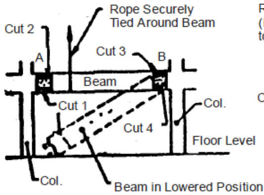
15.3A : R.C. Beams
