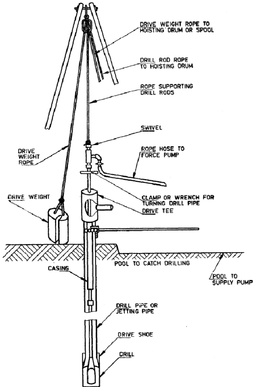
FIG. 23.9 SIMPLE JETTING RIG
