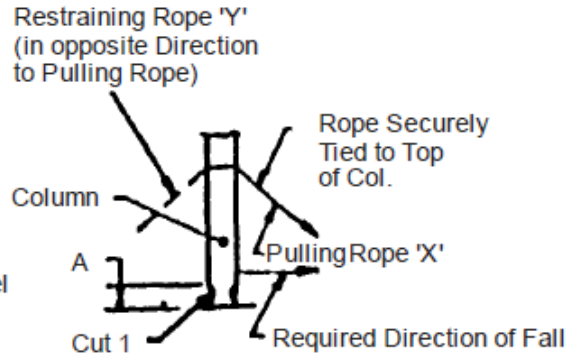
15.3B : R.C. Columns
